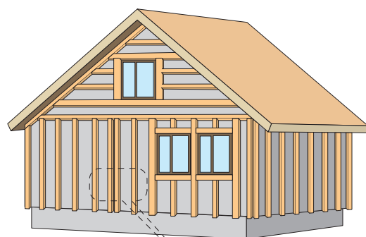
При стыковании сайдинга внахлест, делать «разбежку» стыков
