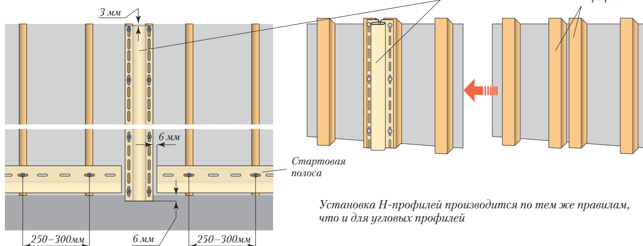
Н-профиль (обязательное применение)
