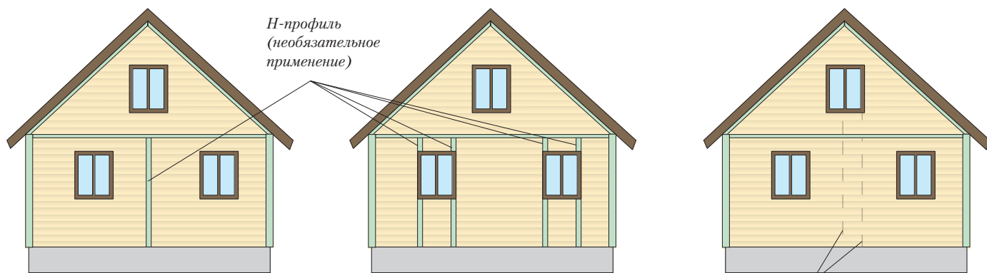
При стыковании сайдинга внахлест, делать «разбежку» стыков
